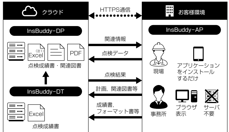
InsBuddyのシステム概要
